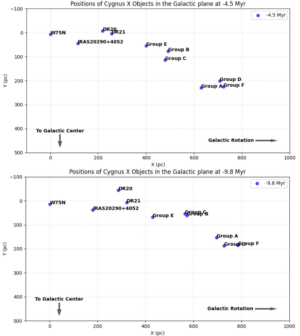
FIGURE 10 – Traceback linéaire sur le plan galactique des objets du Cygne à -4.5 et -9.8 Myr.
